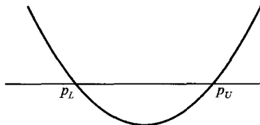
图 6.6.5 二次三项式及其根示意图
