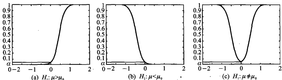
图 7.2.2 g(\mu) 的图形
