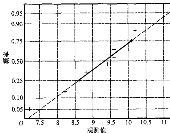
图 7.5.2 例 7.5.1 的正态概率图
