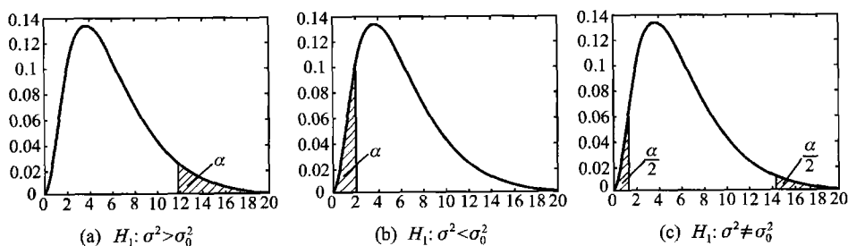
图 7.2.3 三种 \chi^2 检验的拒绝域 ( n-1=6, \alpha=0.05 )
