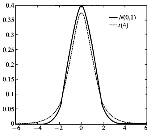
图 5.4.3 t 分布与 N(0,1) 的密度函数
