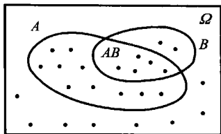
图 1.4.1 例 1.4.2 的维恩图
