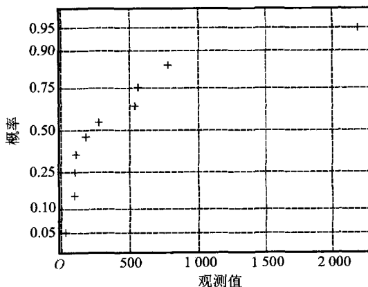
图 7.5.3 例 7.5.2 的正态概率图
