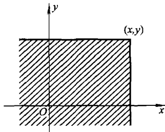
图 3.1.1 以 (x, y) 为顶点的无穷直角区域
