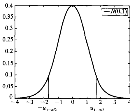
图 6.6.3 标准正态分布示意图
