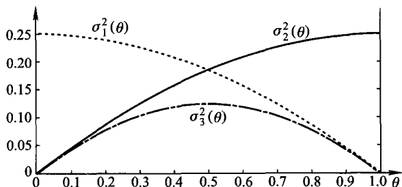
图 6.3.1 三个相合估计的渐近方差的比较
