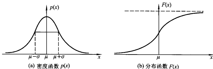
图 2.5.1 正态分布
