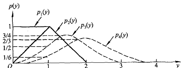
图 4.4.1 均匀分布的卷积
