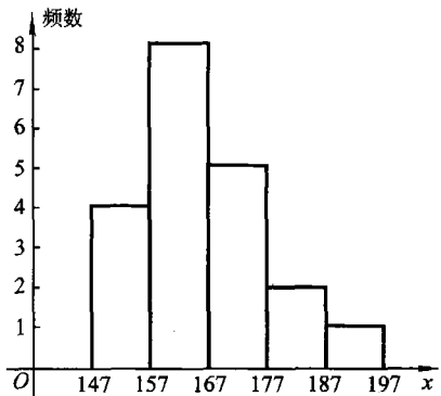
图 5.2.2 例 5.2.2 的频数直方图
