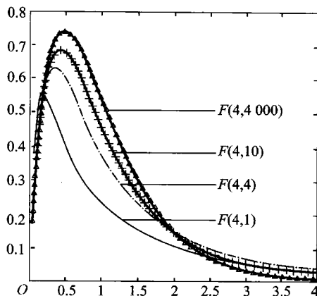
图 5.4.2 F 分布的密度函数
