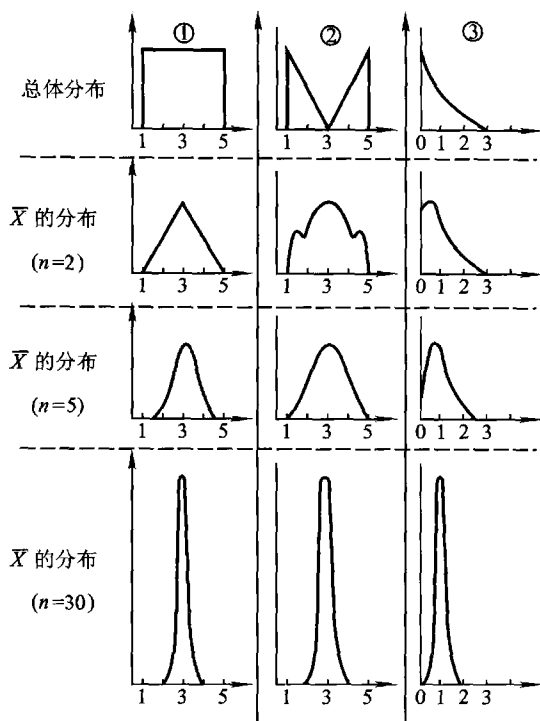
图 5.3.3 不同总体样本均值的分布
