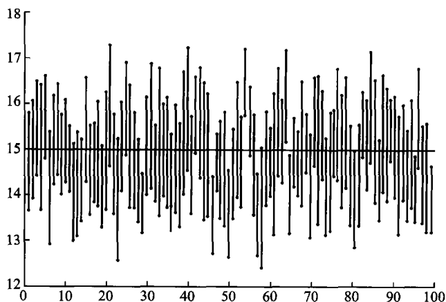
图 6.6.1 \mu 的置信水平为 0.90 的置信区间
