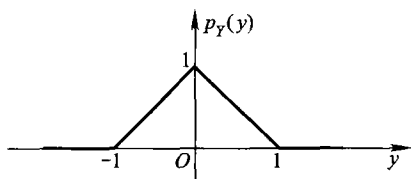
图 3.2.3 Y 的边际密度函数 (三角形分布)
