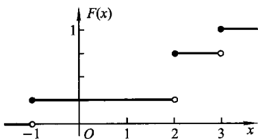
图 2.1.3 离散随机变量的分布函数
