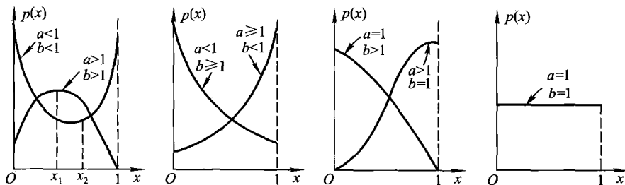
图 2.5.7 贝塔密度函数曲线
