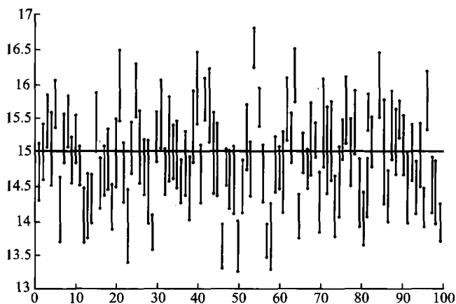
图 6.6.2 \mu 的置信水平为 0.50 的置信区间
