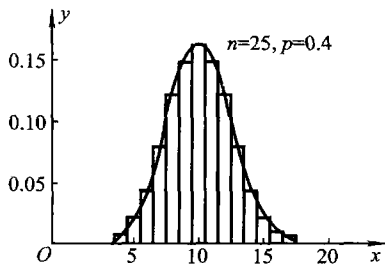
图 4.4.2 二项分布正态近似时的修正
