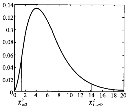
图 6.6.4 \chi^2 分布置信区间示意图
