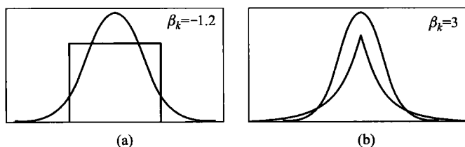
图 2.7.4 两个密度函数与标准正态分布密度函数的比较
