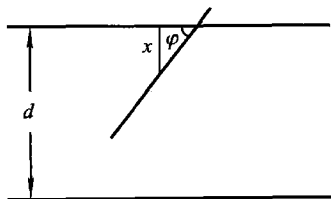
图 1.2.5 蒲丰投针问题
