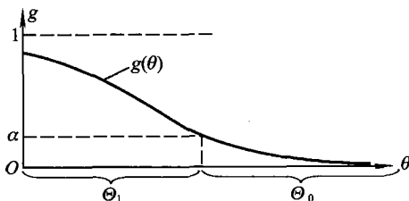
图 7.1.2 例 7.1.2 的势函数 g(\theta)
