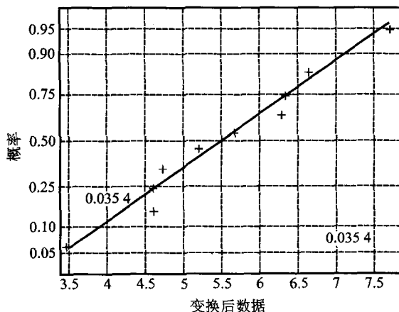
图 7.5.4 变换后数据的正态概率图
