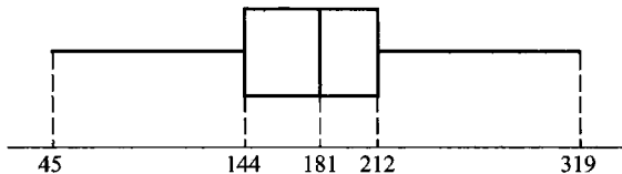
图 5.3.7 月销售量数据的箱线图
