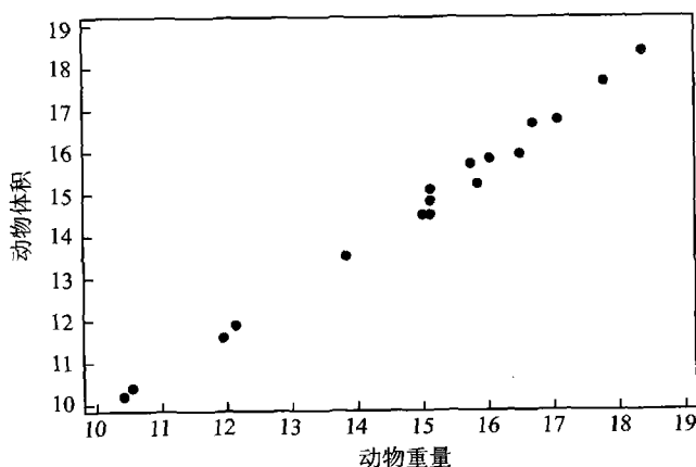
图 8.4.3 动物体积与动物重量的散点图
