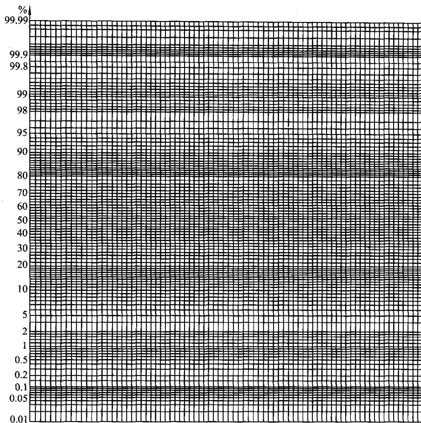
图 7.5.1 正态概率图
