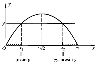
图 2.6.1 y = \sin x 的图形
