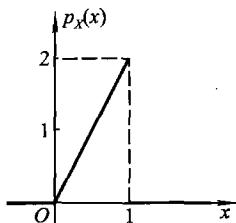
图 3.2.2 X 的边际密度函数 ( Be(2, 1) )
