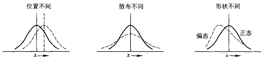
(b) 概率密度函数 p(x) 的不同形状
