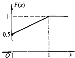
图 2.1.8 既非离散又非连续的分布函数示例
