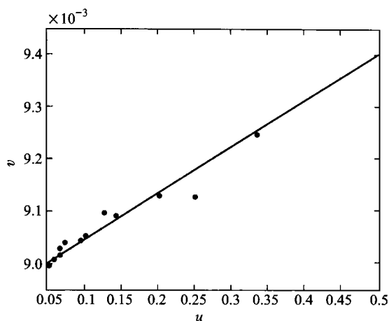
图 8.5.3 变换后数据的散点图
