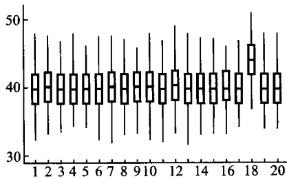
图 5.3.9 20 天生产的某产品的直径的箱线图
