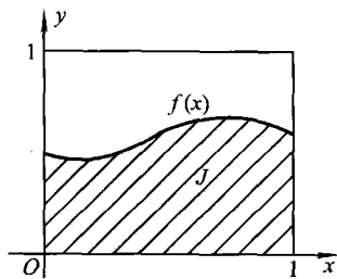
图 4.3.1 随机投点法
