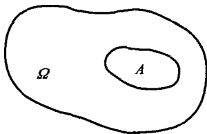
图 1.2.3 几何概率
