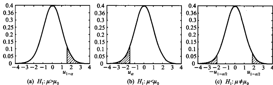
图 7.2.1 u 检验的拒绝域
