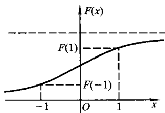
图 2.1.1 柯西分布函数
