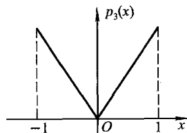
图 2.3.1 比较三个分布的方差与标准差
