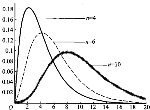
图 5.4.1 \chi^2(n) 分布的密度函数
